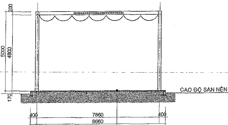
MẶT CẮT 1-1
