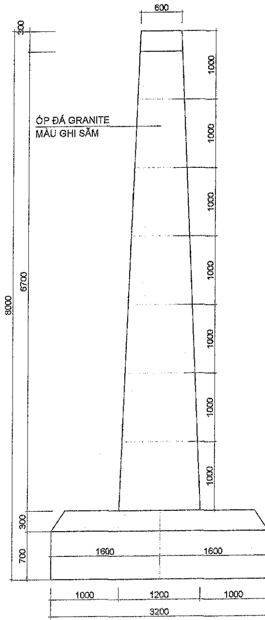
MẶT BÊN
