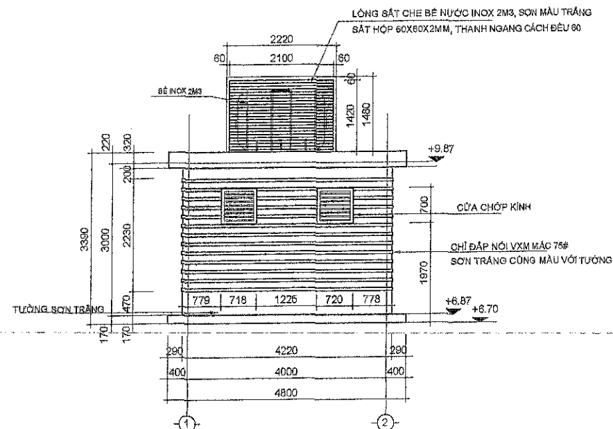
MẶT ĐỨNG TRỰC 1-2
