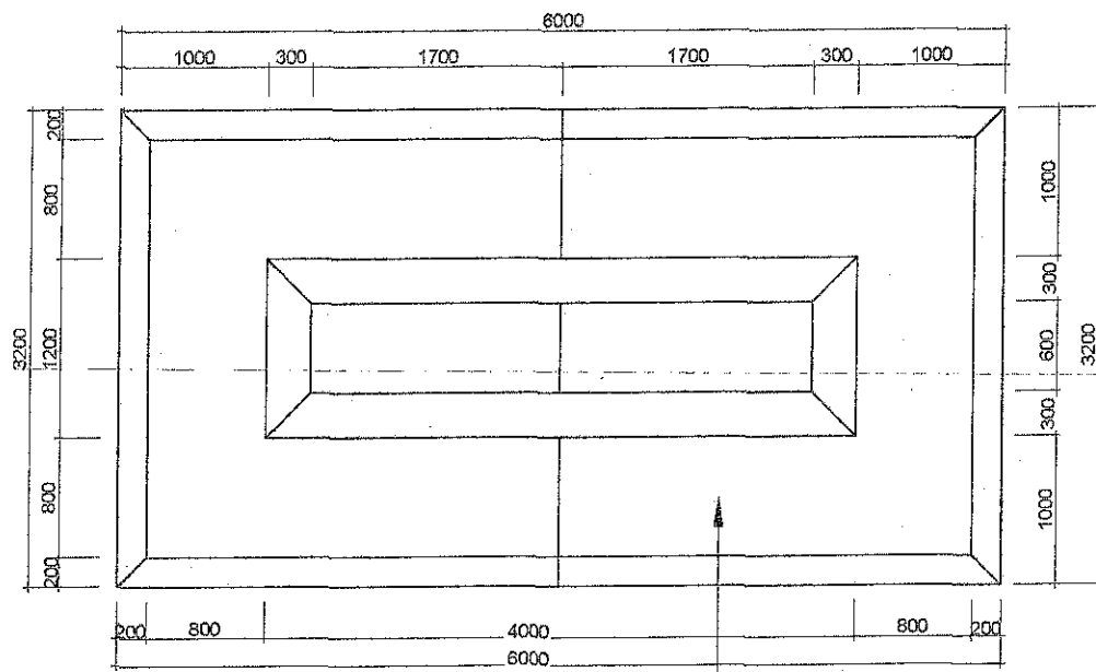
MẶT BẰNG
