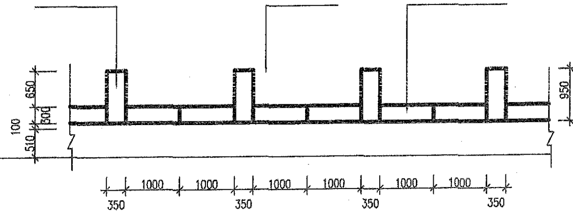
MẶT ĐỨNG LAN CAN BỜ KÈ ĐIỂN HÌNH
