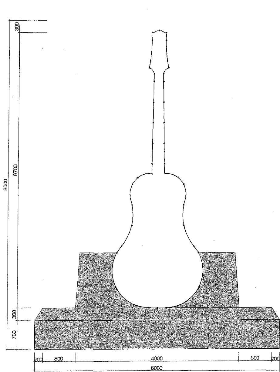
MẶT ĐỨNG CHÍNH
