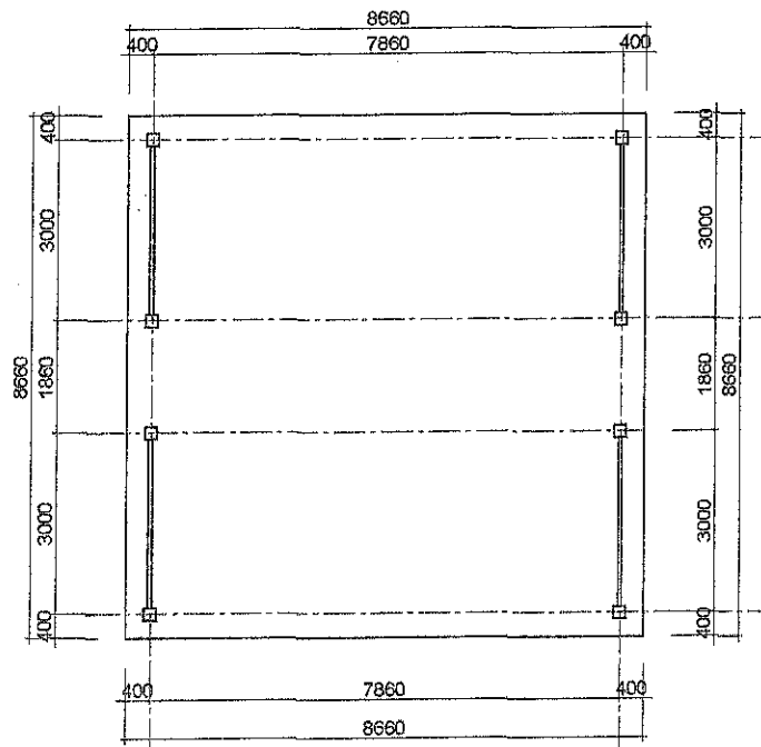
MẶT BẰNG
