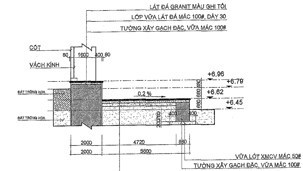
CHI TIẾT TAM CẤP CHÒI
