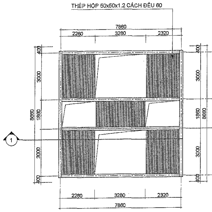
MẶT BẰNG MÁI
