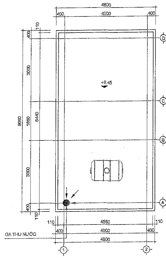
MẶT BẰNG MÁI
