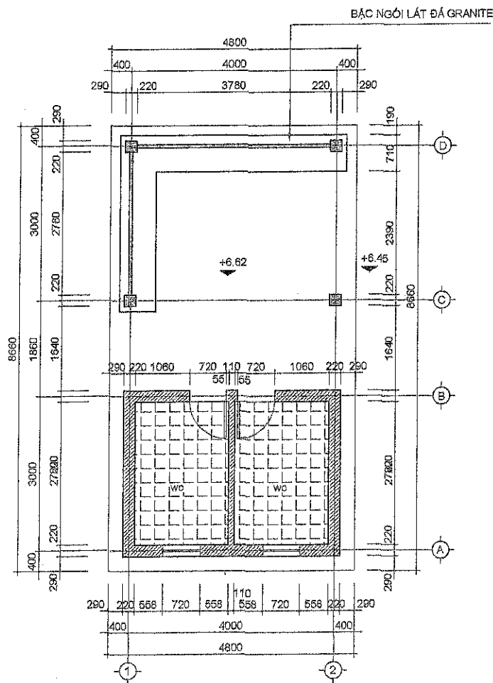
MẶT BẰNG
