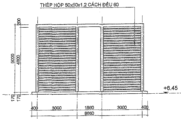
MẶT BÊN
