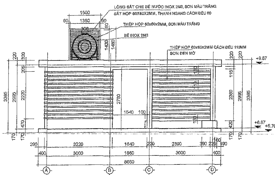
MẶT ĐỨNG TRỰC A-D
