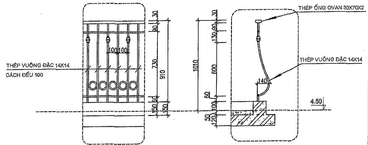
CHI TIẾT LAN CAN SẮT
