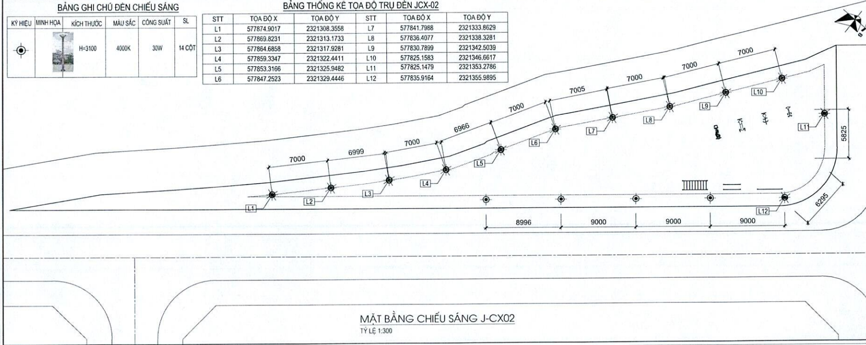
BẢNG THỐNG KÊ TỌA ĐỘ TRỤ ĐÈN JCX-02
