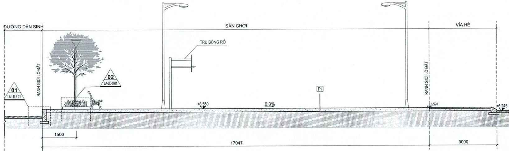
MẶT CẮT 2-2 TỶ LỆ 1:70
