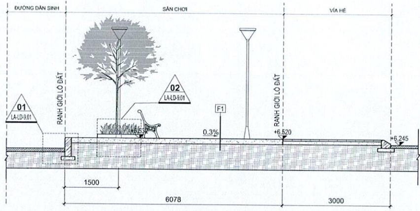
MẶT CẮT 4-4 TỶ LỆ 1:70
