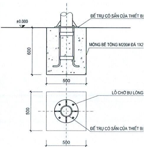
CHI TIẾT LẮP ĐẶT THIẾT BỊ ĐIỂN HÌNH TỶ LỆ 1:20
