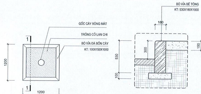
CHI TIẾT 02: MẶT BẰNG BÓN CÂY TỶ LỆ 1:40
