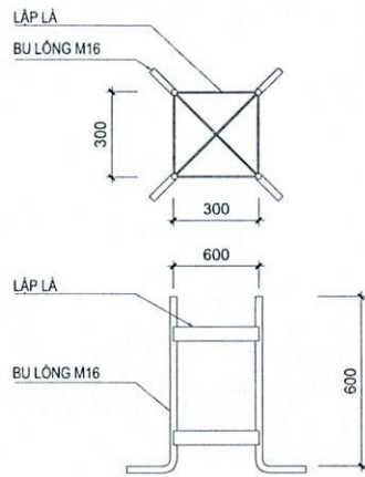
CHI TIẾT KHUNG THÉP MỎNG TỶ LỆ 1:20
