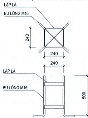
CHI TIẾT KHUNG THÉP MỎNG TỶ LỆ 1:20
