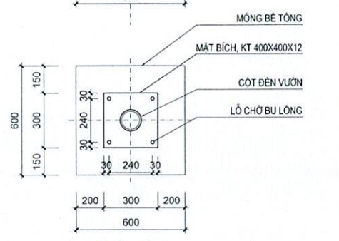
MẶT BÍCH ĐỂ CỘT TỶ LỆ 1:20
