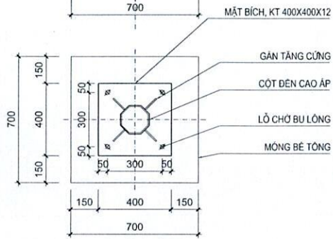
MẶT BÍCH ĐỂ CỘT TỶ LỆ 1:20
