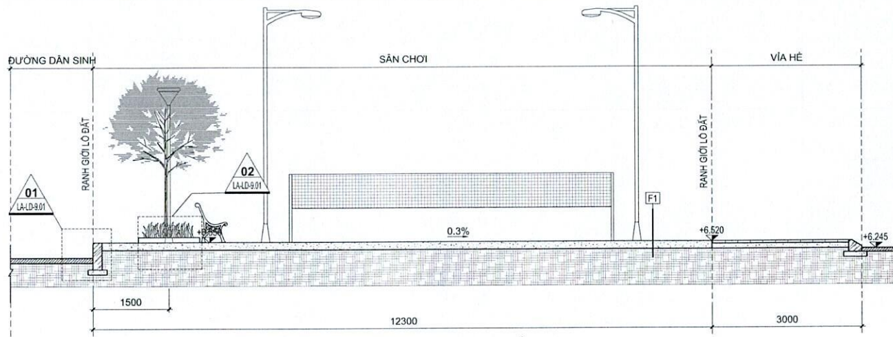
MẶT CẮT 1-1 TỶ LỆ 1:70
