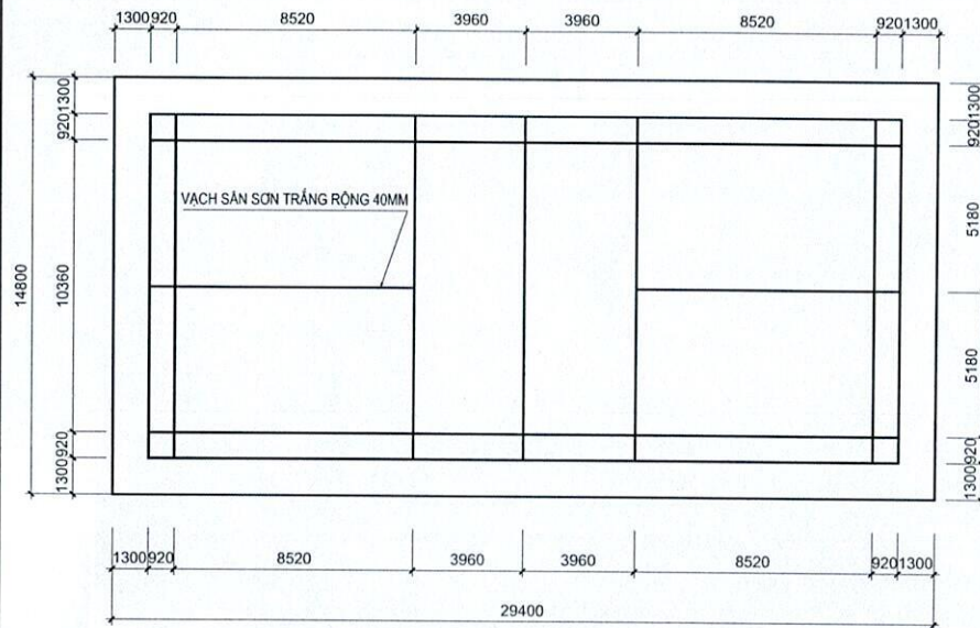
CHI TIẾT KÍCH THƯỚC SÂN CẦU LÔNG TỶ LỆ 1:200
