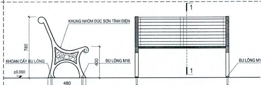
MẶT BÊN GHẾ TỶ LỆ 1:20
