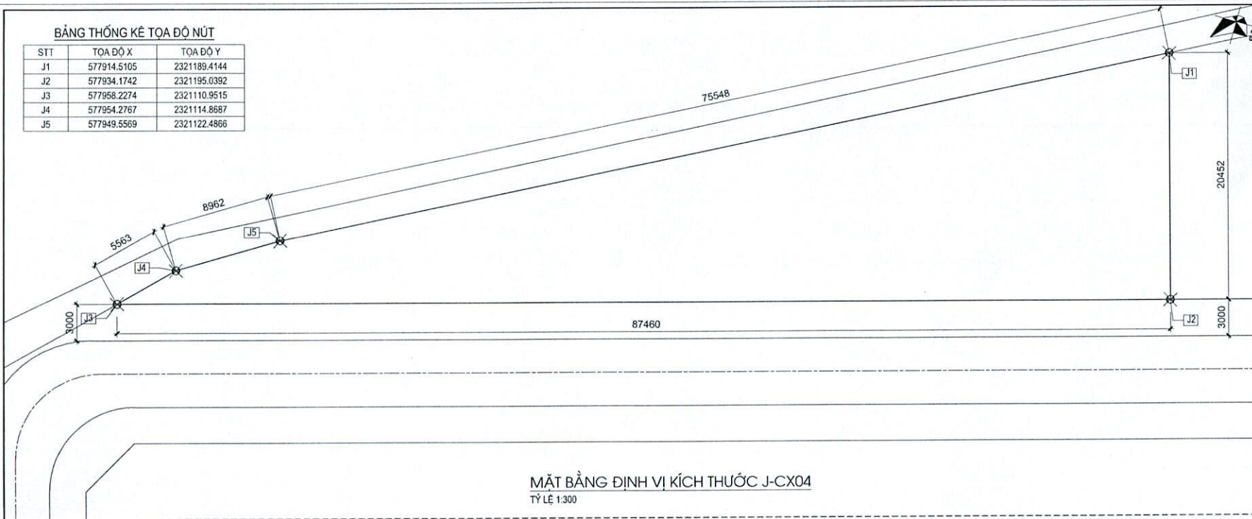
BẢNG THỐNG KÊ TỌA ĐỘ NÚT
