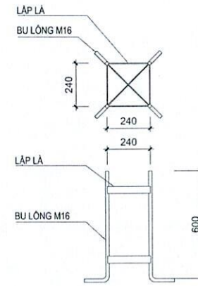
CHI TIẾT KHUNG THÉP MỎNG TỶ LỆ 1:20
