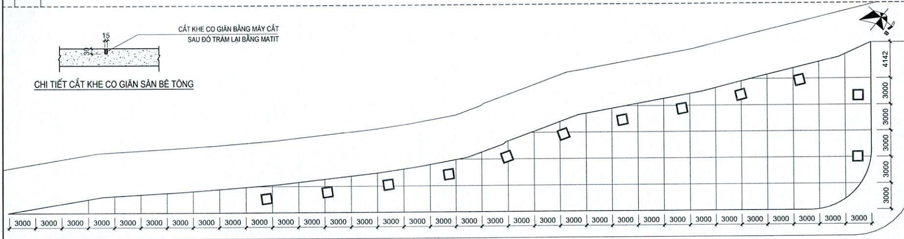
MẶT BẰNG KHE CO GIẢN SÀN BÊ TÔNG J-CX04 TỶ LỆ 1:300
