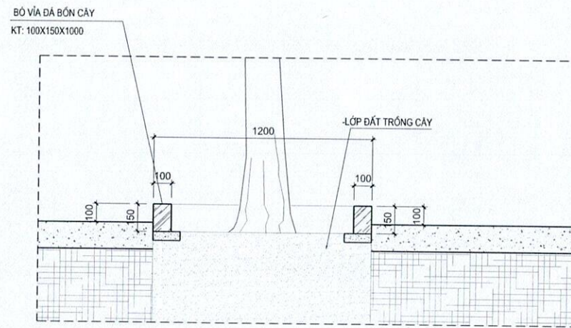
CHI TIẾT 02: MẶT CẮT 1-1 TỶ LỆ 1:20
