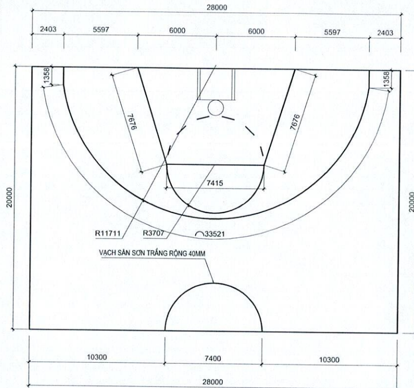
CHI TIẾT KÍCH THƯỚC SÂN BÓNG RỎ TỶ LỆ 1:200
