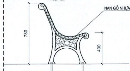
MẶT BÊN GHẾ TỶ LỆ 1:20
