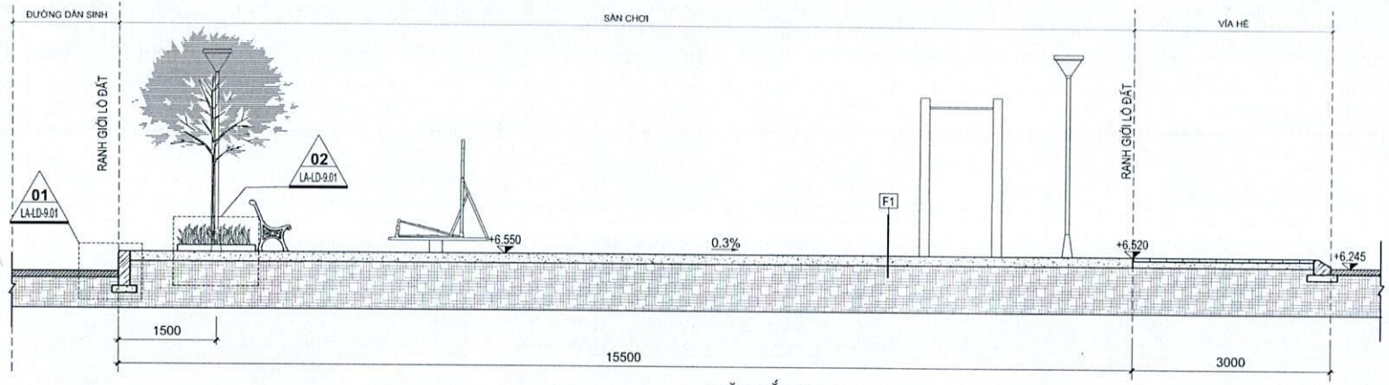
MẶT CẮT 3-3 TỶ LỆ 1:70
