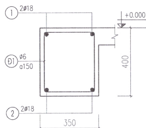
DẦM D2-1A (SL : 01, L=2800MM)
