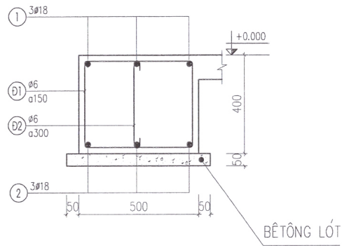
DẦM D2-8 (SL : 01, L=1460MM)
