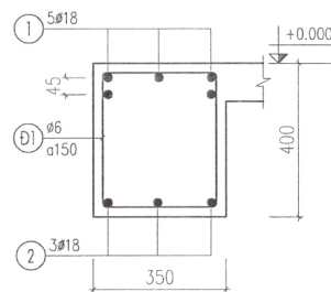
DẦM D2-3 (SL : 01, L=4310MM)
