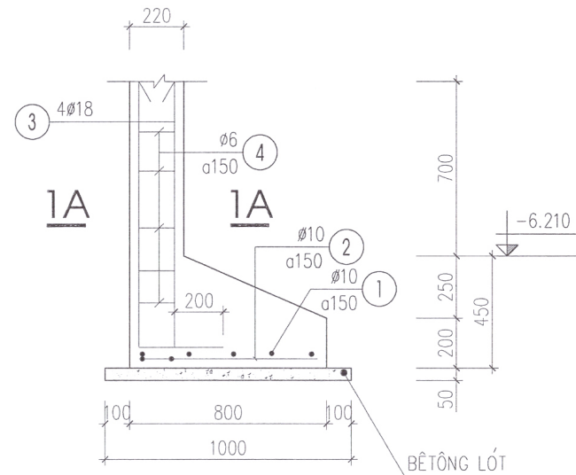
MẶT CẮT 1 - 1
