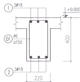
DẦM D2-5 (SL : 04, L=6000MM)
