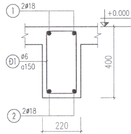
DẦM D2-2 (SL : 01, L=10310MM)
