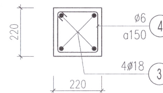
MẶT CẮT 1A- 1A
