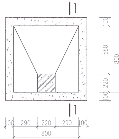
MÓNG MĐ1 (SL : 06)
