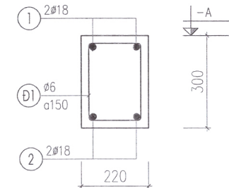
DẦM D1-1(SL: 01, L=14045MM)
